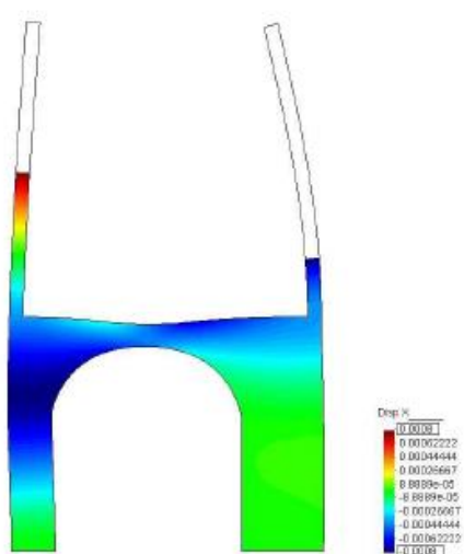
Figura. 7 Deformacions i desplaçament en X estat actual
