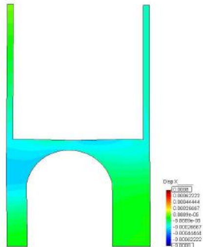
Figura. 8 Deformacions i desplaçament en X projecte
